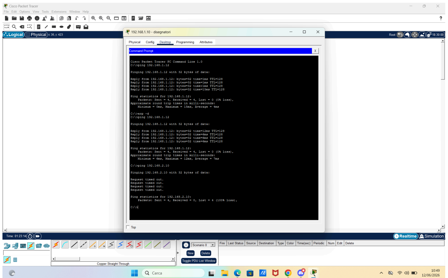
Figura 3 Ping fallito tra host appartenenti a Vlan differenti
